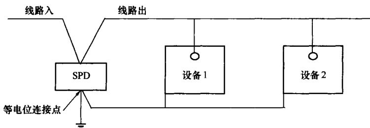
图 11 凯文接线法
