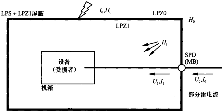
(b) 采用 LPZ1 空间屏蔽和 LPZ1 入口 SPD 防护的 LPMS
