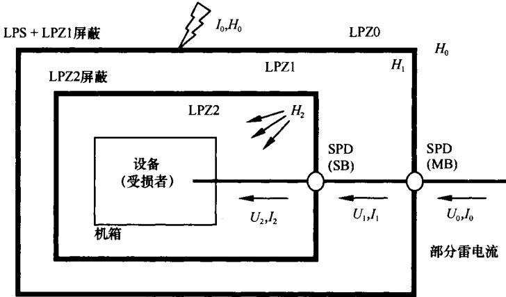
(a) 采用空间屏蔽和“协调配合的 SPD 防护”的 LPMS
