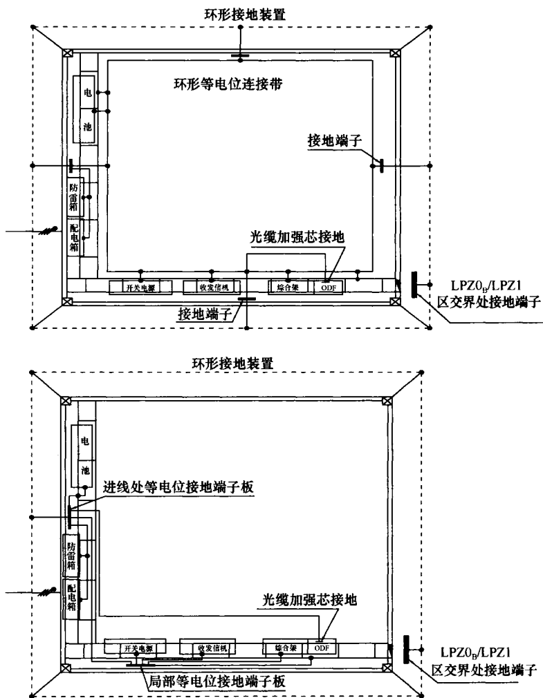
图 15 移动通信基站的接地
