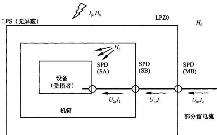
图 4 LEMP 防护措施系统 (LPMS) 示例 (二)
