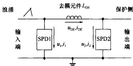
图 13 SPD 能量配合电路模型
