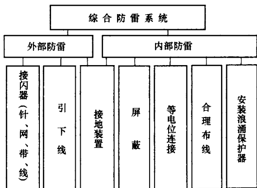
图1 建筑物电子信息系统综合防雷框图
