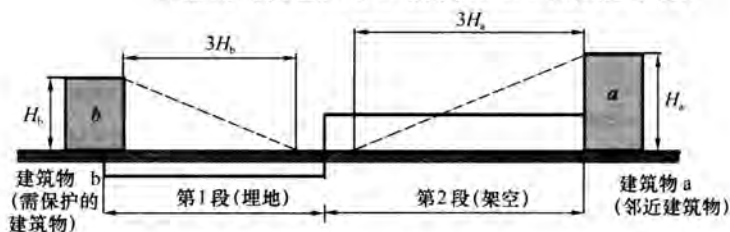
图 B. 5. 5 线路两端的建筑物
