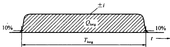
图 C.0.1-3 长时间雷击波形参数
