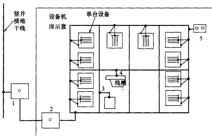
(b) M型等电位连接网络
