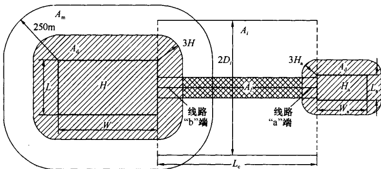
图 B.5.6 截收面积 ( A_d, A_m, A_i, A_l )
